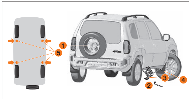
Рис. 80. Подъем автомобиля при замене колёс
