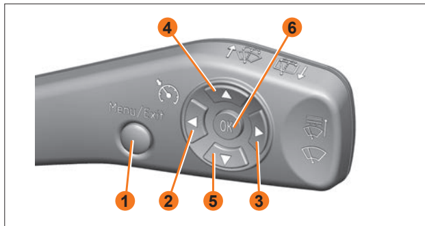
Рис. 41д. Клавиши управления круиз-контролем и ограничителем скорости
