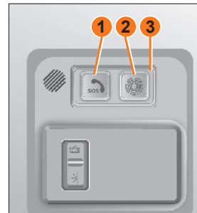
Рис. 70. Компоненты БИП (в вариантном исполнении)
