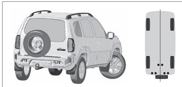
Рис. 34. ТСУ и точки его крепления (в варианном исполнении)
