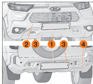
Рис. 63. Крепление номерных знаков
