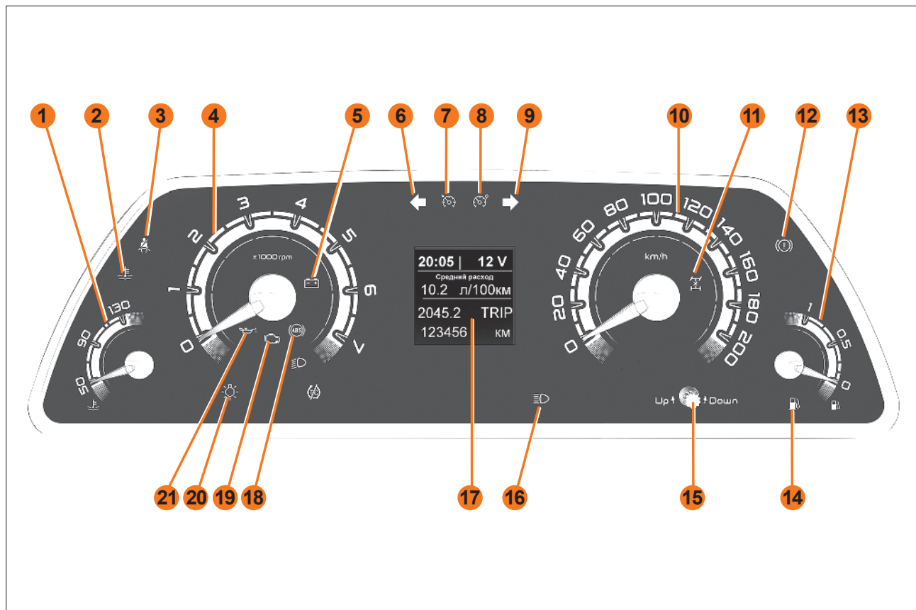
Рис. 41а. Комбинация приборов
