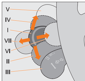
Рис. 44. Подрулевые переключатели
