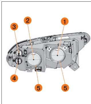
Рис. 82. Блок-фара
