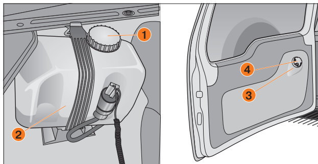
Рис. 78. Бачки омывателей стёкол
