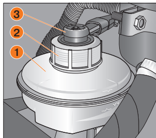
Рис. 73. Проверка уровня тормозной жидкости
