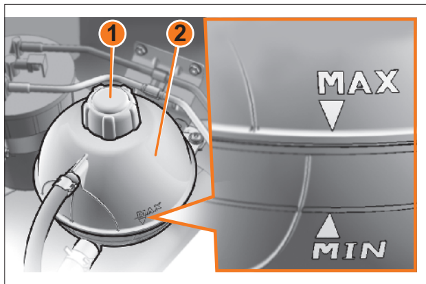
Рис. 72. Проверка уровня охлаждающей жидкости в расширительном бачке
