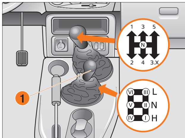
Рис. 48. Положение рычагов трансмиссии
