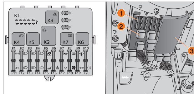
Рис. 81. Монтажный блок – схема установки
