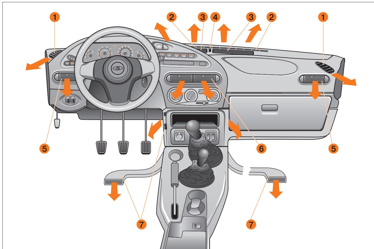
Рис. 49. Распределение потоков воздуха системы вентиляции и отопления салона
