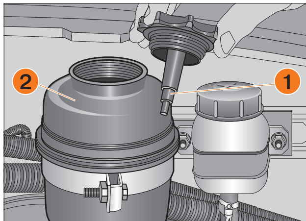
Рис. 75а. Бачок гидроусилителя руля (в вариантном исполнении)
