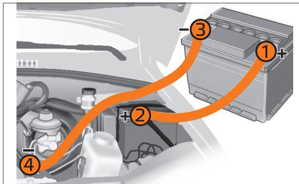
Рис. 64. Схема подключения пусковых проводов к вспомогательной батарее
