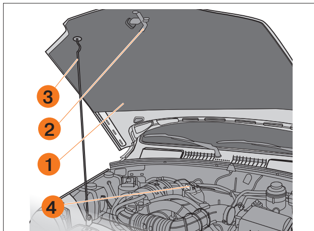
Рис. 37. Открывание капота
