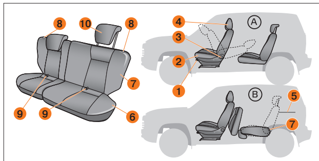
Рис. 11. Сиденья (в вариантном исполнении)
