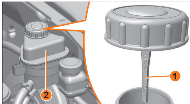
Рис. 75б. Бачок гидроусилителя руля (в вариантном исполнении)
