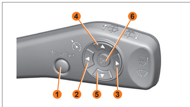
Рис. 41г. Переключатель стеклоочистителя с шестью клавишами управления
