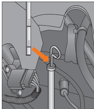
Рис. 71. Проверка уровня масла в картере двигателя
