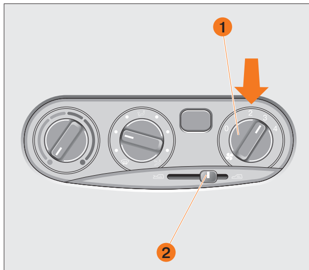
Рис. 52. Правый вращающийся переключатель
